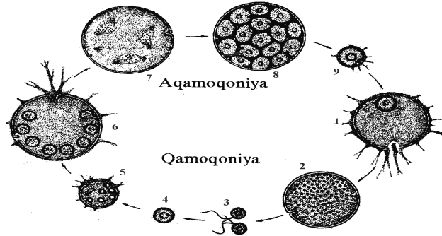
Şəkil 4. Myxotheca arenilega foraminiferasının inkişaf tsikli (Qrelə görə): 1 – birnövəli qamont, 2 – qamətlərin əmələ gəlməsi (qamoqoniya), 3 – qamətlərin kopulyasiyası, 4 – ziqota, 5 – cavan aqamont, 6 – böyüyən aqamont, 7 – meyoza (reduksiya vaxtı), 8 – aqamətin əmələ gəlməsi (aqamoqoniya), 9 – cavan aqamətlər (qamont)
