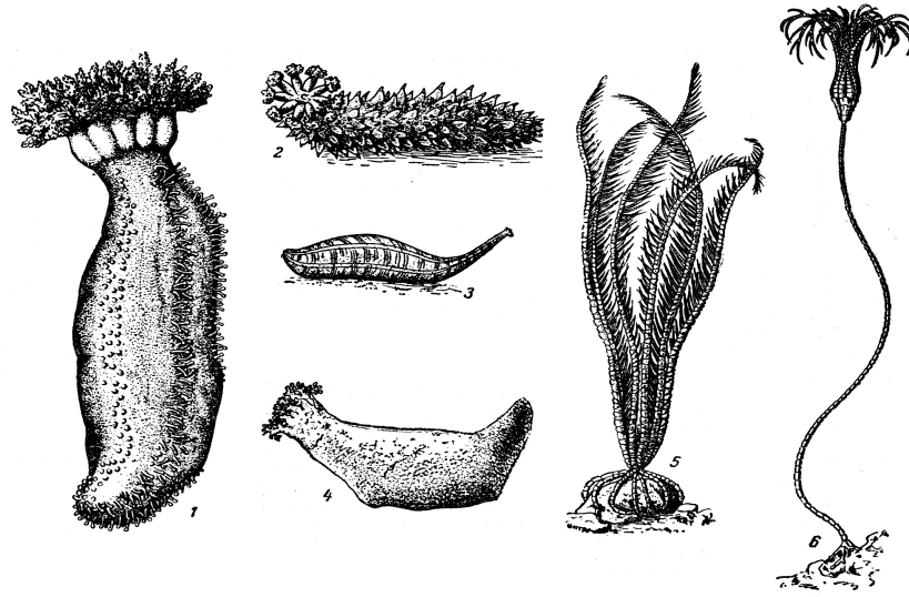
Şəkil 214. Holoturilər və dəniz zanbaqları (Abrikosovdan): 1 – şimal dənizlərində rast gəlinən Cucumaria frondosa dəniz xiyarı, 2 – Yapon dənizində rast gəlinən trepanq ( Stichopus japonicum ), 3 – ayaqsız holoturi, Caudina (Yapon dənizi), 4 – şimal dənizlərində məskunlaşan dəniz toyuğu ( Psolus phantapus ), 5 – adi dəniz zanbağı ( Heliometra glacialis ), 6 – Kars dənizində rast gəlinən saplaqlı dəniz zanbağı ( Bothryocrinus decadactylus )
