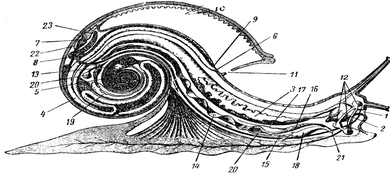
Şəkil 160. Tənək ilbizi Helix pomatia (sxematik quruluşu): 1 – ağız, 2 – udlaq, 3 – tüpürcək vəziləri, 4 – bağırsağ, 5 – qaraciyər, 6 – anal dəliyi, 7 – ürək, 8 – böyrək, 9 – böyrəyin xarici dəliyi, 10 – ağciyər, 11 – nəfəslik, 12 – udlaqətrafi qanqli, 13 – hermafrodit vəzi, 14 – toxum-yumurta borusu, 15 – yumurta borusu, 16 – toxum borusu, 17 – flaqullum (qaytan), 18 – «sevgi oxları» və ya «hövr» kisəsi, 19 – zülal vəzisi, 20 – toxumqəbuledici rezervuarı və axarı, 21 – cinsi dəlik, 22 – perikardial boşluq, 23 – renoperikardial dəlik (oxlarla qanın hərəkət istiqaməti göstərilir)
