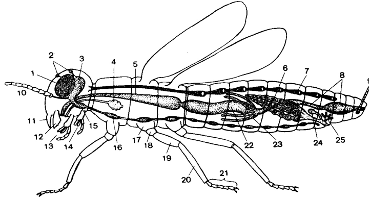
Şəkil 99. Qanadlı həşəratın quruluş sxemi (Xadorna görə): 1 – mürəkkəb göz, 2 – sadə gözcük, 3 – beyin, 4 – tüpürcək vəzisi, 5 – ön bağırsağ, 6 – yumurtalıq, 7 – ürək, 8 – arxa bağırsağ, 9 – serkilər (quyruq qılıçları), 10 – antennalar, 11 – üst dodaq, 12 – mandibula, 13 – 14 – birinci və ikinci maksillalar, 15 – udlaqaltı qanqlı, 16 – qarın sinir zənciri, 17 – çanaq, 18 – burma, 19 – bud, 20 – baldır, 21 – pəncə, 22 – orta bağırsağ, 23 – malpigi boruları, 24 – toxumqəbuledici, 25 – əlavə cinsi vəzilər
