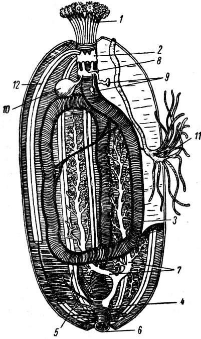
Şəkil 215. Ayaqsız holoturinin daxili quruluşu: 1 – çuxıntılı tac, 2 – udlaqətrafi kirəcli halqa, 3 – bağırmaq, 4 – kloaka, 5 – küvyerə açılan küvyer vəzisi, 6 – anal dəlik, 7 – bağırmaq ağciyərləri (su ağciyərləri), 8 – ambulakral sistemin həlqəvi kanalı, 9 – daşlı kanal, 10 – poliev qovuğu, 11 – qonada, 12 – boylama əzələ lifləri
