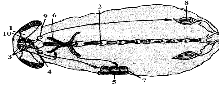
Şəkil 114. Həşərat bədənində əsas endokrin və hədəf orqanların yerləşməsi (Novaka görə): 1 – beyin, 2 – döş və qarıncıq qanqlilərinin neyrosekretor hüceyrələri, 3 – beyinin neyrosekretor hüceyrələri, 4 – udlaqaltı qanqlinin neyrosekretor hüceyrələri, 5 – örtüklər, 6 – protorakal vəzilər, 7 – hipodermal hüceyrələr, 8 – yumurtalıqlar, 9 – əlavə cisimlər ( corpora allata ), 10 – kardial cisimlər ( corpora cardiaca ); oxlarla həşəratın inkişafının tənzimlənməsi zamanı hormonların hədəf orqanlarına təsiri göstərilir
