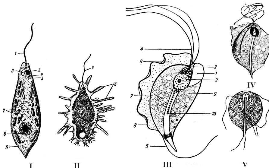
Şəkil 6. Qamçılıların müxtəlif formaları. I - Euglena viridis (Dofleyne görə: 1 - qamçı, 2 - stiqa, 3 - rezervuar, 4 - yığılıb-açılan vakuol, 5 - yığıcı vakuollar, 6 - paramil dənələri, 7 - xromatoforlar, 8 - nüvə); II - Mastigamoeba aspera (Şultsə görə: 1 - qamçılar, 2 - psevdopodilər); III - Trichomonas angusta (1 - sitostom, 2 - bazal cisimcik (kinetosoma), 3 - nüvə, 4 - ön qamçılar, 5 - arxa qamçı, 6 - undulyar (titrək) membrana, 7 - onun bazal fibrili, 8 - kənar lif, 9 - vakuollar, 10 - aksostil); IV - Trichomonas hominis ; V - Lamblia intestinalis
