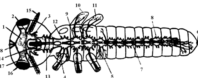
Şəkil 112. Həşəratın mərkəzi sinir sistemi (1 – protoserebrum, 2 – rıncıq seqmentləri sinirləri, qanqlisi, 9 – ortadöş qanql udlaqaltı qanqlisi, 14 – tritosererebrumun qanqlisi, 17 – beyinin optik sahəsi, 18 –
