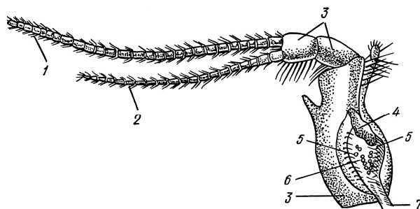
Şəkil 61. Çay xərçənginin antennulası (Şimkeviçə görə): 1 – 2 – bığcıqın iki qamçısı, 3 – əsas buğumlar, 4 – statosist çuxurunun dəliyi, 5 – statosistin dibində yerləşən hissi tükcüklər, 6 – statosistin daxilindəki kristal dənəciklər, 7 – sinir. Hər iki qamçı lamisə və qoxu tükcükləri ilə örtülüdür.
