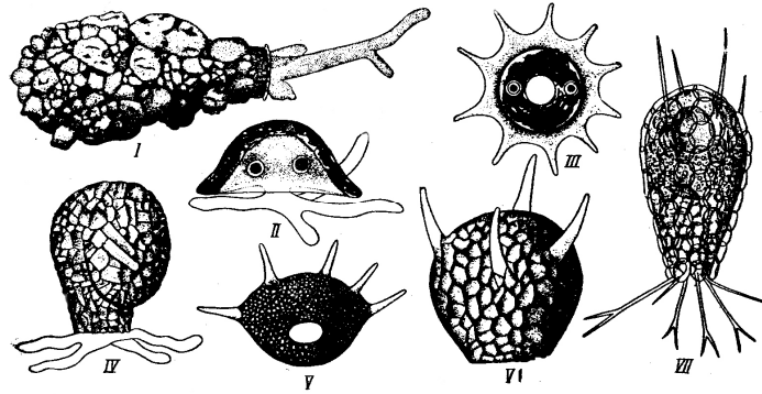
Şəkil 3. Çanaqlı kökayaqların müxtəlif növləri. I.- Diffugia pyriformis ; II – Arcella vulgaris ; III – Arcella dentata ; IV - Lesquereusia modesta ; V – Centropyxis ; VI – Diffugia corona ; VII – Euglypha alveolata
