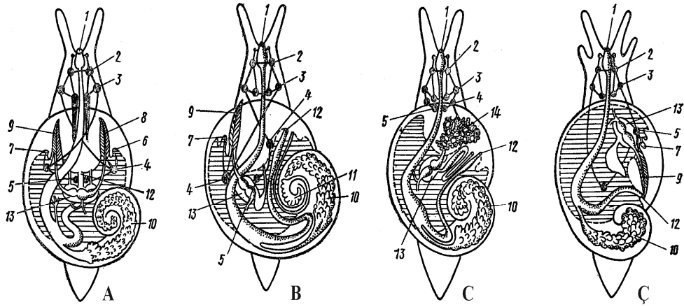
Şəkil 163. Müxtəlif qarnıayaqlı molyuskaların quruluş sxemi (Ştəmpələ görə): A, B – önqəlsəməlilər, C – ağciyərlilər, Ç – arxaqəlsəməlilər: 1 – ağız, 2 – serebral qanqli, 3 – plevral qanqli, 4 – parietal qanqli, 5 – visseral qanqli, 6, 7 – osfradilər, 8, 9- ktenidilər, 10 – qaraciyər, 11 – cinsi vəzi, 12 – anus, 13 – perikardium, 14 – ağciyərin damarlı toru
