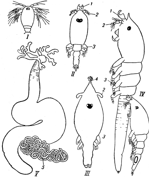
Şəkil 69. Parazitlik edən kürəkayaqlı xərçəng Lernaeocera –nın metamorfozu (Averintsevə görə): I – metanauplius, II – kapepod sürfə, III –oturaq sürfə mərhələsi, IV – cütləşmə, V - yetkin dişi fərd: 1 – antennula, 2 – antenna, 3 – döş ətrafları, 4 – paraziti sahibə birləşdirən yapışma orqanı, 5 – yumurta qaytanı
