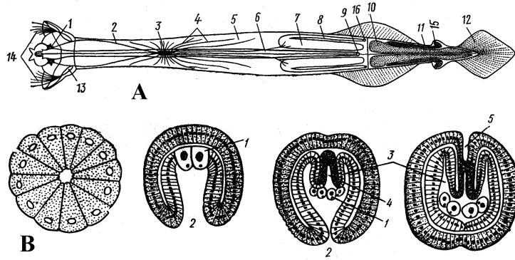
Şəkil 224. Sagitta gazellae ( Chaetognatha ) qılçənəlisinin quruluşu və inkişafı: A - qarın tərəfdən görünüşü (Delyaja görə): 1 – beyin, 2 – udlaqətrafi konnektiv, 3 – qarın qanqlisi, 4 – sinirlər, 5 – selom, 6 – bağırsaq, 7 – yumurtalıq, 8 – yumurta borusu, 9 – anus, 10 – toxumluq, 11 – toxum borusu, 12 – quyruq üzgəci, 13 – baş vəzisi, 14 – xitin qarmaq-qılıçlar, 15 – erkək cinsi dəlik, 16 – diş cinsi dəlik; B – inkişafının dörd mərhələsi (Hertviqə görə): 1 – ilkin cinsi hüceyrələr, 2 – blastopor, 3 – selomun rüşeymi (enterosel üsulla), 4 – bağırsaq, 5 – ikinci ağız
