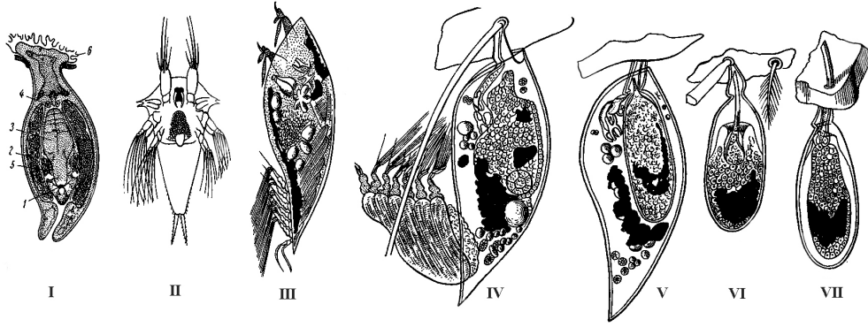
Şəkil 71. Sacculina . I – yetkin parazitin köndələn kəsiyi, II- nauplius, III – si- pris-sürfə, IV, V, VI, VII- sahibin bıçığına birləşdikdən sonra parazitə sonrakı inkişaf mərhələləri: 1 – sinir düyünü, 2 – mantiya daxilində yumurtalar kütləsi, 3 – yu- murtalıq, 4 – toxumluq, 5 – əlavə cinsi vəzi, 6 – kökşəkilli çıxıntılar
