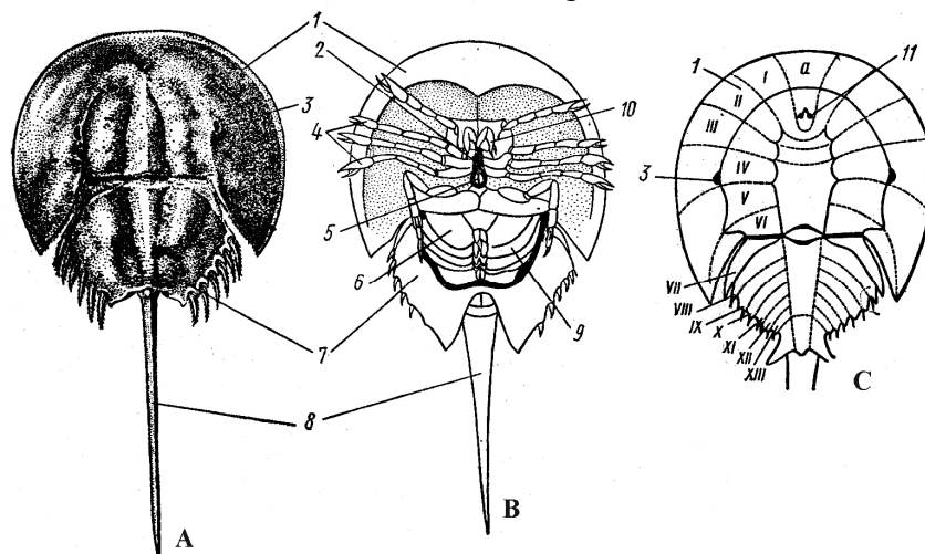
Şəkil 77. Limulus polyphemus nizəquyruğun quruluşu: A – bel tərəfdən görünüşü (Van der Hovenə görə), B – qarın tərəfdən görünüşü (Snodgrassa görə), C – buğumlaşmanın sxemi (İvanova görə): 1 – başdöş qalxanı, 2 – ağız, 3 – mürəkkəb gözlər, 4 – gözici ətraflar, 5 – xilərilər, 6 – qəlsəmə qapağı, 7 – qarın şöbəsi, 8 – quyruq nizəsi, 9 – qəlsəmə daşıyan ətraflar, 10 – xeliserlər, 11 – tək gözcüklər, I-XIII – sərhədləri qırıq xətlərlə göstərilən seqmentlər, a – akron
