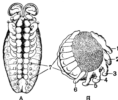
Şəkil 87. Hürümçəkkimilərdə rüşeymin inkişafı (Nataliyə görə): A – əqrəb rüşeyminin qarın tərəfdən görünüşü; B – hürümçək rüşeyminin yan tərəfdən görünüşü: 1 – xeliserin rüşeymi, 2 – pedipalplar, 3 – 6 – gəzici ətrafların rüşeymləri, 7 – qarıncıq ətraflarının rüşeymi
