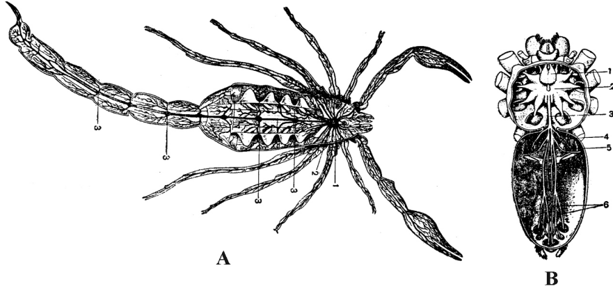
Şəkil 86. Hörmüçəkkimilərin sinir sistemi: A – əqrəbin sinir sistemi: 1 – baş beyin, 2 – udlaqaltı düyün, 3 – qarın sinir zəncirinin düyünləri; B – ev hörmüçəyi Tegetaria –nın sinir sistemi: 1 – baş beyin, 2 – baş-döş və qarıncıq düyünlərinin birləşməsindən əmələ gələn udlaqaltı düyün, 3 – qarın sinir sütunu, 4 – qarın sütununun şaxələri, 5 – ağciyər, 6 – tor ziyillərin sinirləri
