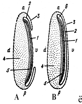
Şəkil 126. Həşəratda rüşeym qatlarının formalaşması (Heydərə görə): A və B – inkişafın iki ardıcıl mərhələləri: 1 – rüşeym zolağı, 2 – amnion, 3 – seroz, 4 – sarılıq, 5 – entoderma və mezodermanın ümumi rüşeymi (entomezoderma), 6 – amniotik boşluq, a – ön, p – arxa, qütb, d – bel, v – ventral (qarın tərəf)
