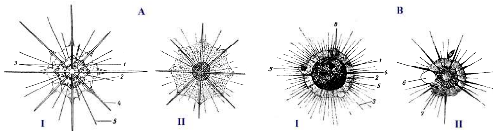
Şəkil 5. Radiolariyaların (A) və Günəşkimilərin (B) müxtəlif formaları.
