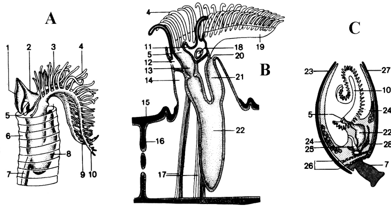
Şəkil 217. Üçbuğumlu heyvanların ( Trimera ) quruluş xüsusiyyətləri (De-lage, Herouard; Cori; Brien → görə): A – qanadqəlsəməli Rhabdopleura ( Pterobranchia ); B – briozoy Plumatella ; C – çiyinayaqlılar Brachiopoda ( Tentaculata ): 1 – borucuqlu hərəkətməyə xidmət edən protosomanın ventral diski, 2 – mezosoma, 3 – lofoforun daxili səthində yerləşən qidalanma şırımı, 4 – çıxıntı, 5 – ağız dəliyi, 6 – borucuq, 7 – saplaq, 8 – metasoma, 9 – çıxıntıları daşıyan sağ və sol (10) qollar, 11 – epistom, 12 – mezosel, 13 – ön bağırsağ, 14 – metasel, 15 – sistidin kutikulası, 16 – qonşu sistidləri bir-birindən təcrid edən arakəsmə, 17 – retraktor-əzələ, 18 – mezosomda olan qanlı, 19 – lofofor, 20 – anus, 21 – arxa bağırsağ, 22 – mədə, 23 – çanağın ventral qapağı, 24 – yumurtalıqlar, 25 – metanefridi, 26 – qapayıcı və açıcı əzələlər, 27 – çanağın dorsal qapağı, 28 - ürək
