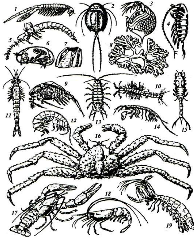
Şəkil 52. Xərçəngkimilər. 1 – qəlsəməayaq ( Branchipus stagnalis ), 2 – qalxancıqlı ( Triops cancriformis ), 3 – su birəsi ( Daphnia pulex ), 4 - kalanus ( Falanus ), 5 – mistakokarid ( Derocheilocaris remanei ), 6 – çanaqlı xərçəng ostrakoda ( Heterocypris reptans ), 7 – dəniz qozası balyanus ( Balanus hammeri ), 8 – parazitik kisədöş xərçəng ( Dendrogaster dichotomus ), 9 – nazikzirehli xərçəng ( Nebalia geoffroyi ), 10 – batinela, 11 – mizid xərçəng ( Mysis relicta ), 12- göl yanüzən xərçəngi ( Gammarus lacustris ), 13 – dəniz ulağı ( Asselus aquaticus ), 14 – qısqacdı ulaq, 15 – kum xərçəng ( Lamprops corroensis ), 16 – kamçatka yengəci ( Paralithoides cameschatica ), 17 – çay xərçəngi ( Potamobius astacus ), 18 – adi krevetka ( Crangon crangon ), 19 – dəvədəllək xərçəng ( Squilla oratoria )
